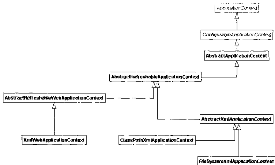
图 5-2 ApplicationContext 接口及其实现
