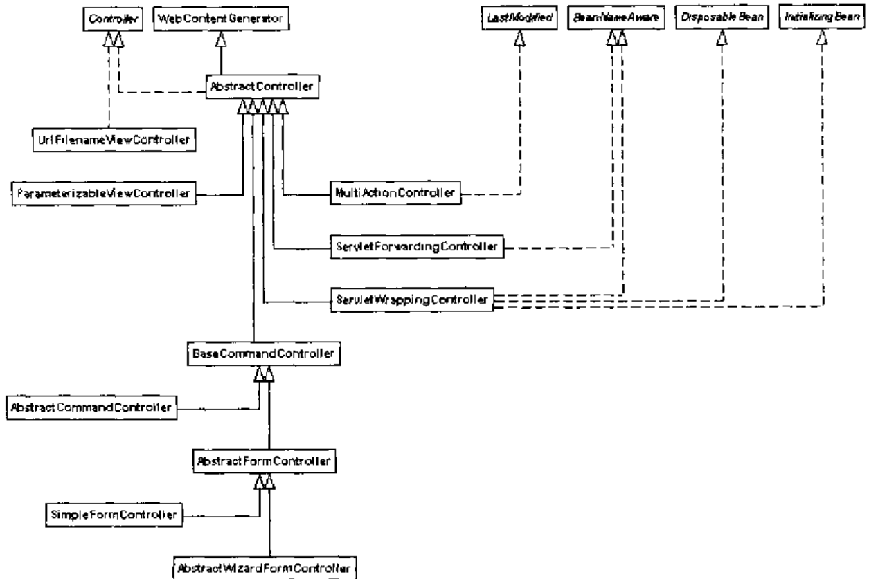
图 14-2 Controller 接口及其实现
