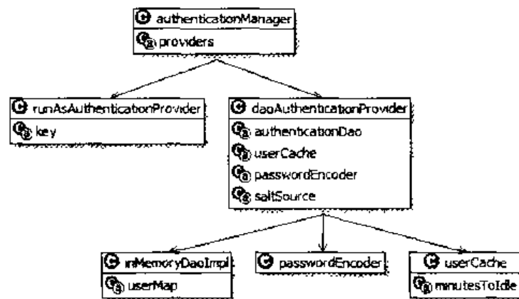
图 17-17 “authenticationManager”的图形式表示
