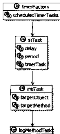
图 12-6 example23 中 appcontext.xml 的 JavaBean 结构
