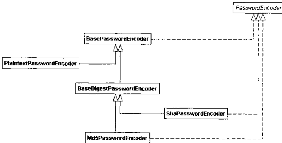
图 17-26 PasswordEncoder 接口及其子类
