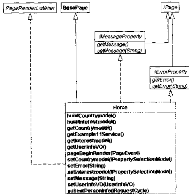
图 5-16 基于 Tapestry 的 UML 类图 (1)
