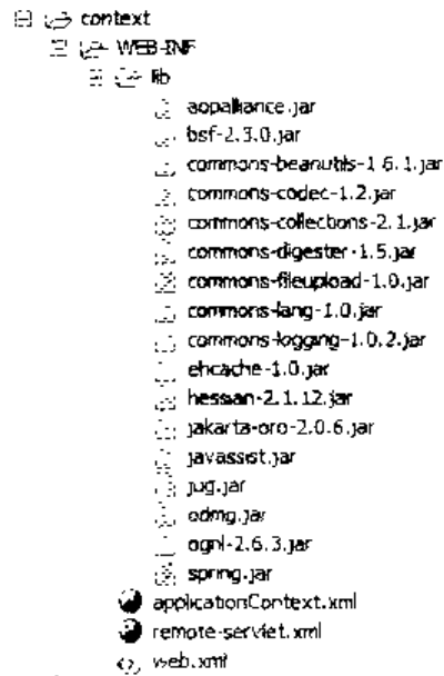
图 13-5 example25.war 使用到的 jar 库
