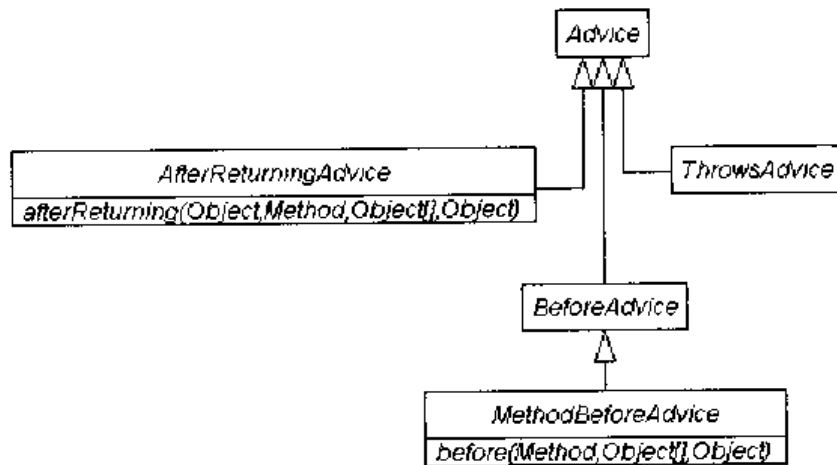
图 4-2 Advice 及相关接口的关系
