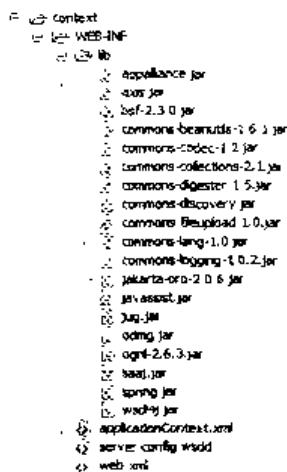
图 13-12 example28.war 使用到的 jar 库
