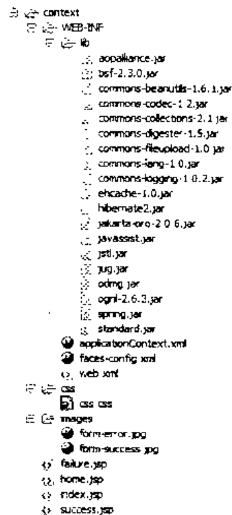
图 16-2 example29 JSF Web 应用结构
