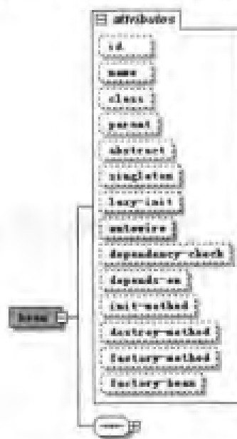
图 B-2 bean 节点的属性
