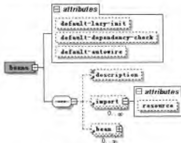
图 B-1 beans 节点的内容模型
