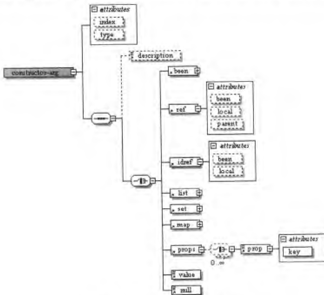
图 B-4 constructor-arg 节点的内容模型
