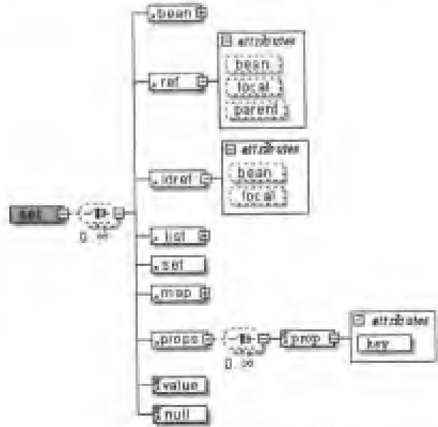
图 B-6 set 节点的内容模型
