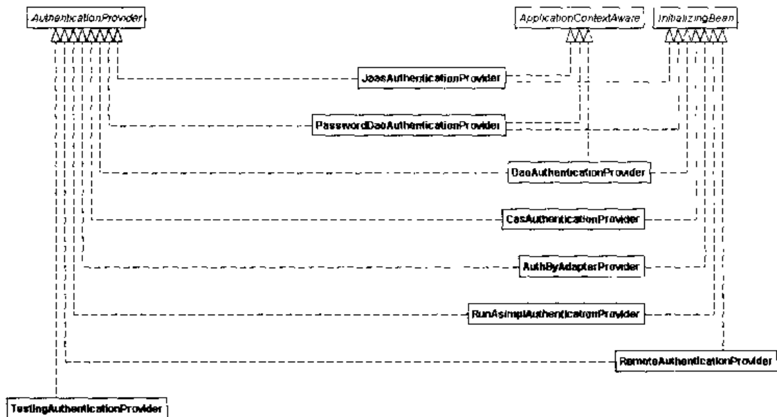
图 17-15 AuthenticationProvider 接口及其子类
