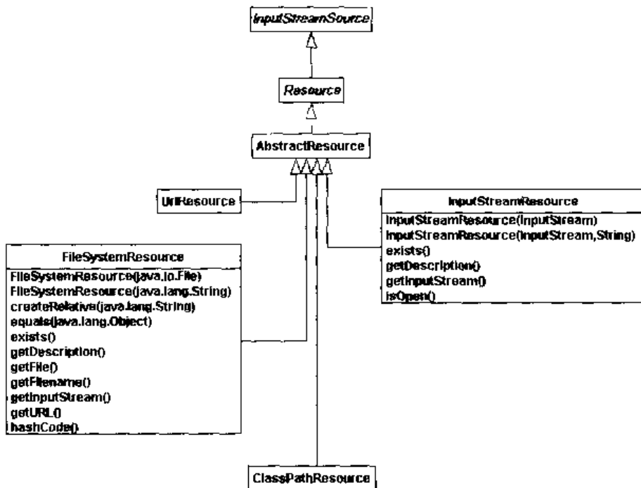
图 1-1 core.io 包所含类的类图
