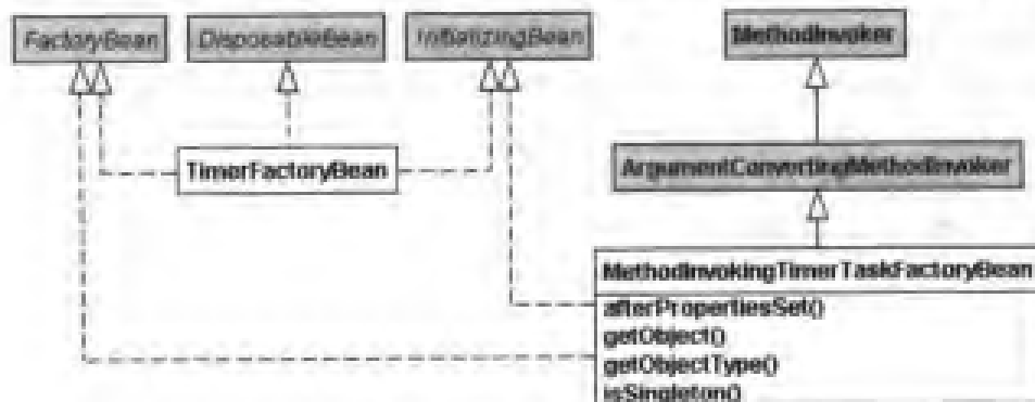
图 12-4 timer 包的类图
