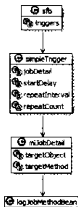
图 12-3 example21 中 appcontextmethod.xml 的 JavaBean 结构
