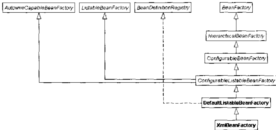
图 3-1 BeanFactory 及其实现
