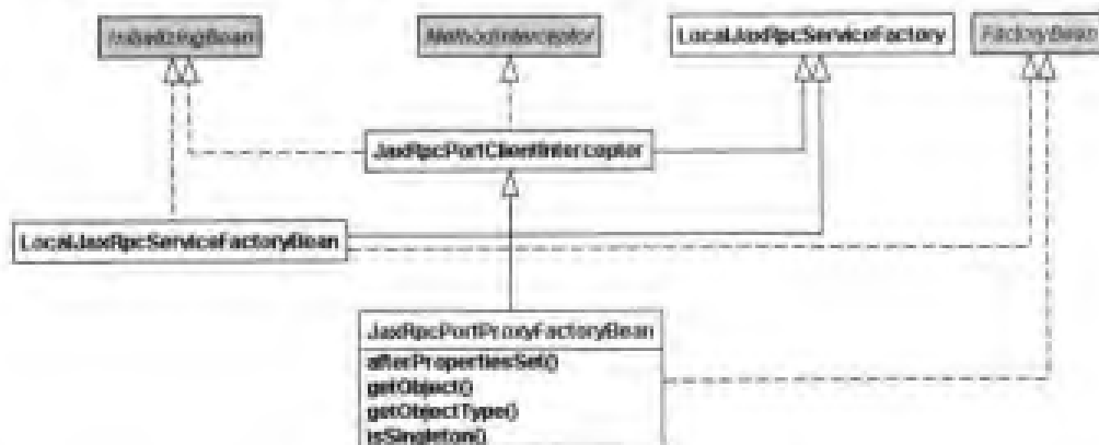
图 13-14 提供 Web 服务的类图
