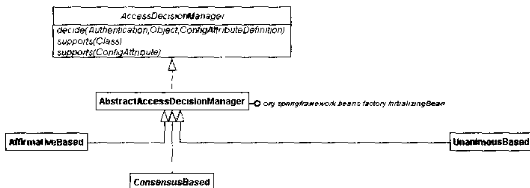
图 17-18 AccessDecisionManager 接口及其子类
