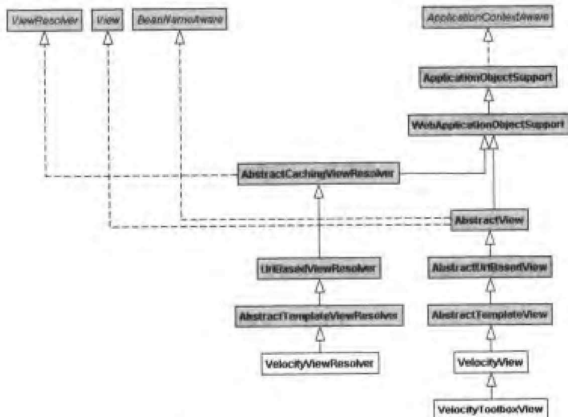
图 14-6 Spring 用于集成 Velocity 的类
