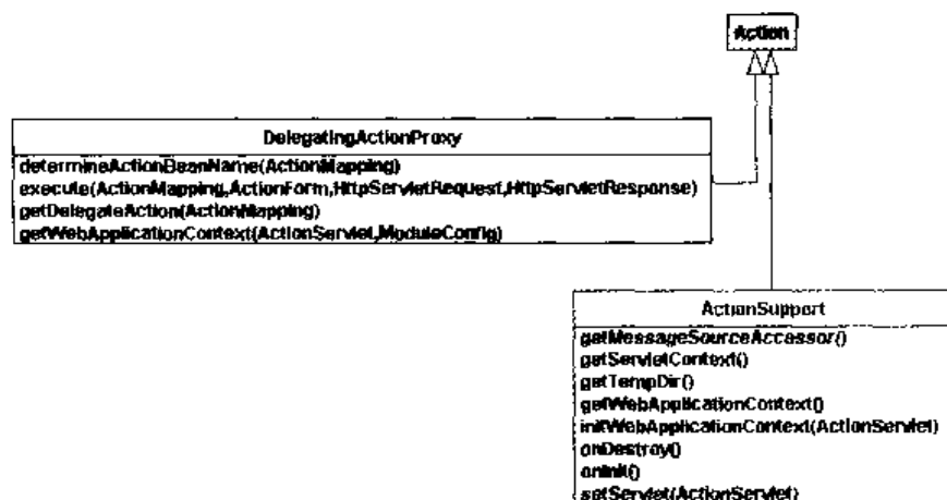
图 14-5 Spring 用于集成 Struts 的 ActionSupport 和 DelegatesActionProxy 类
