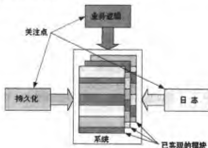
图 4-1 从 AOP Aspect 看待系统 1
