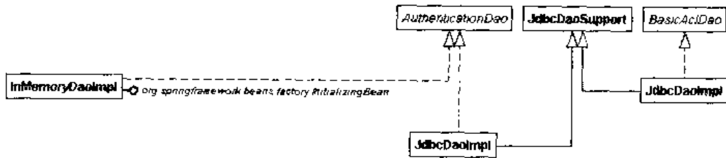
图 17-16 AuthenticationDao 接口及其子类
