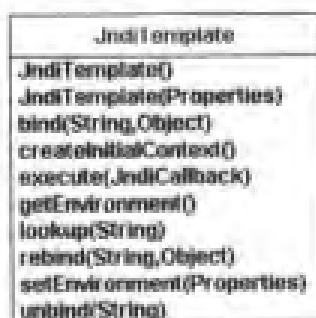
图 6-2 JndiTemplate 类图
