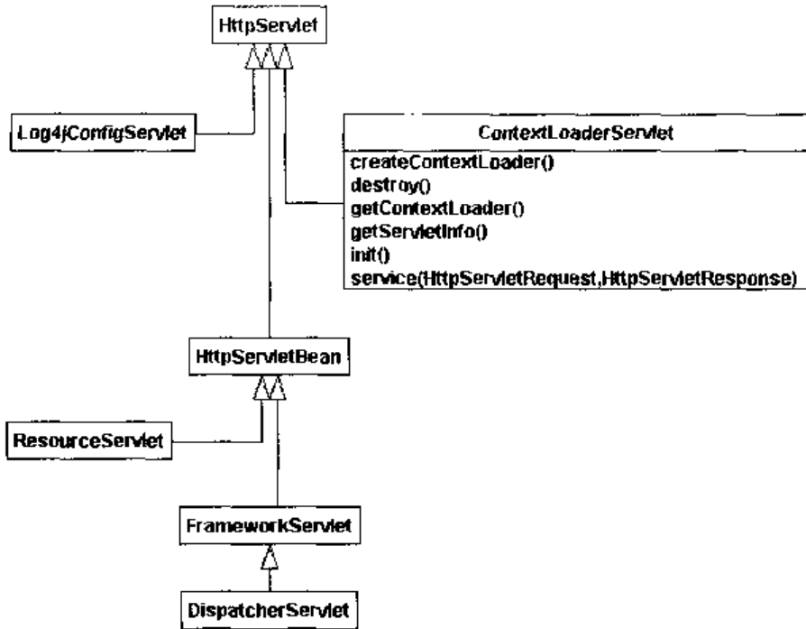
图 3-4 ContextLoaderServlet 类图
