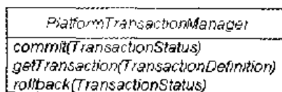
图 7-1 PlatformTransactionManager 接口
