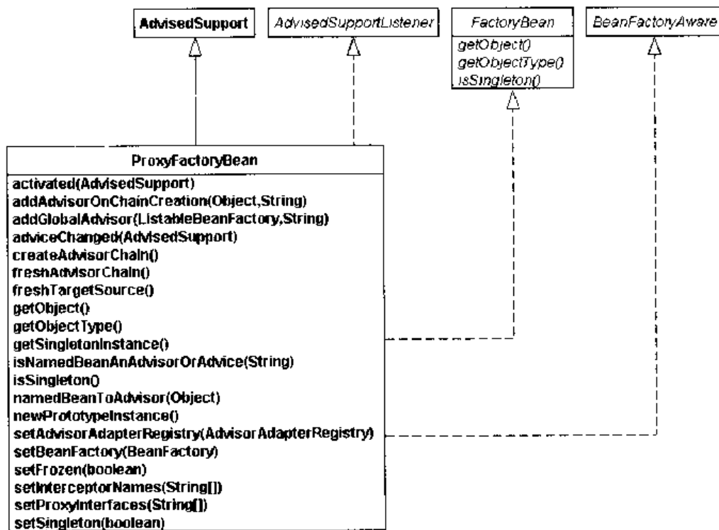
图 4-5 ProxyFactoryBean 类图
