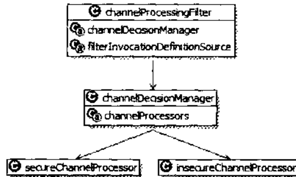
图 17-22 channelProcessingFilter 过滤器
