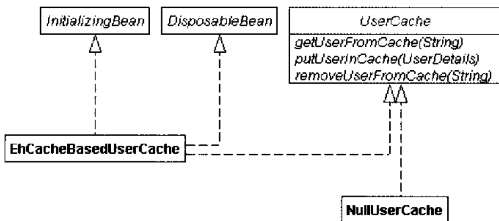
图 17-27 UserCache 接口及其子类
