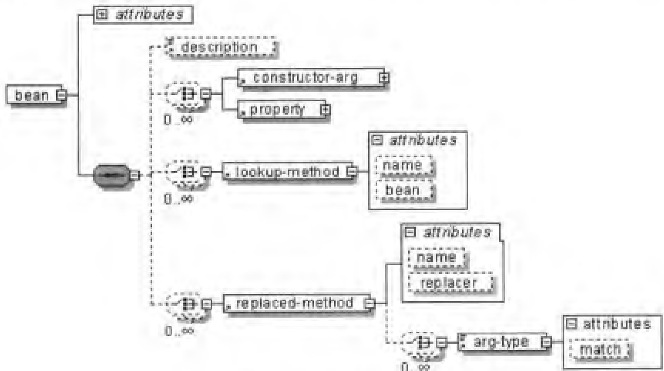
图 B-3 beans 节点的内容模型
