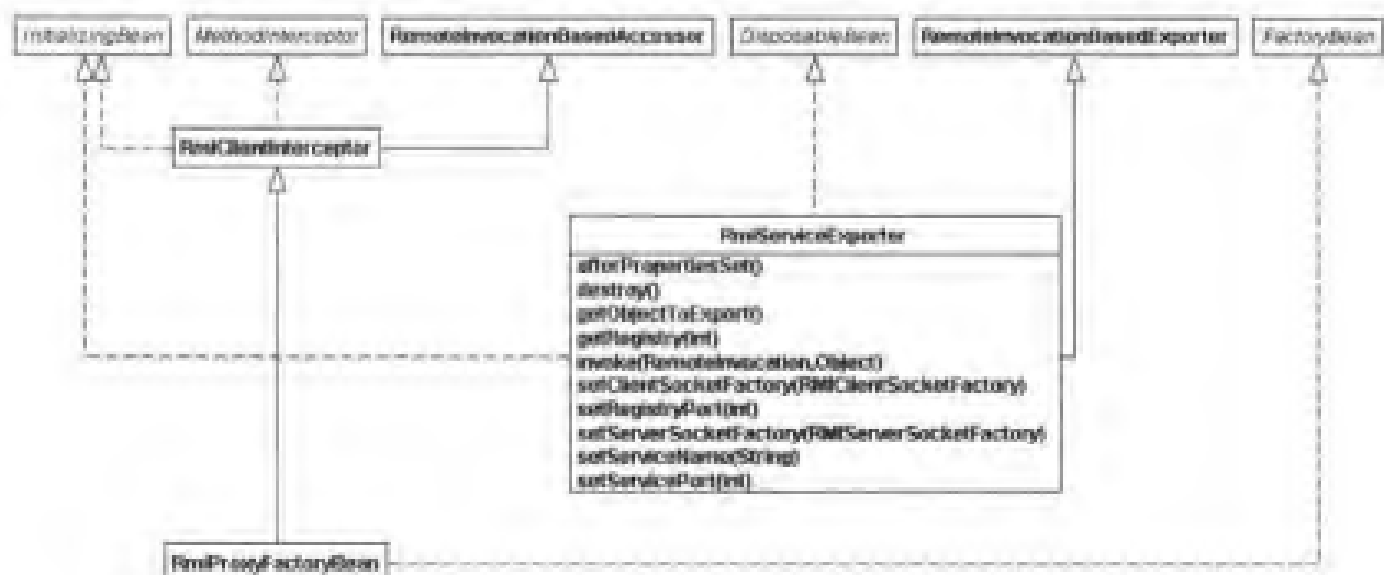
图 13-3 提供 RMI 使能服务的类图
