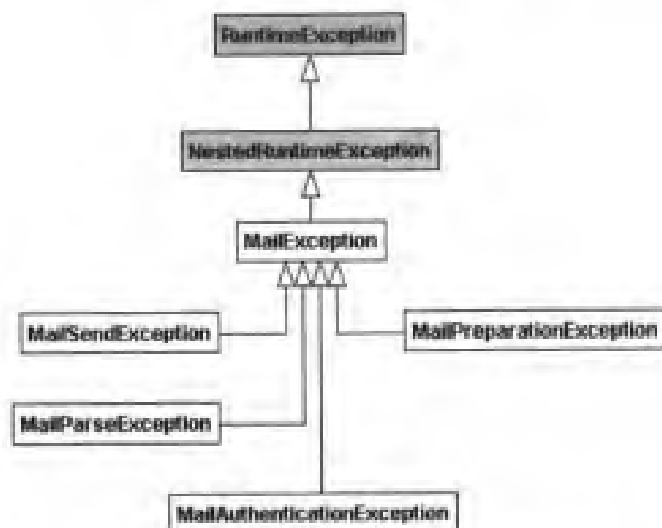
图 9-1 org.springframework.mail 包提供的异常类
