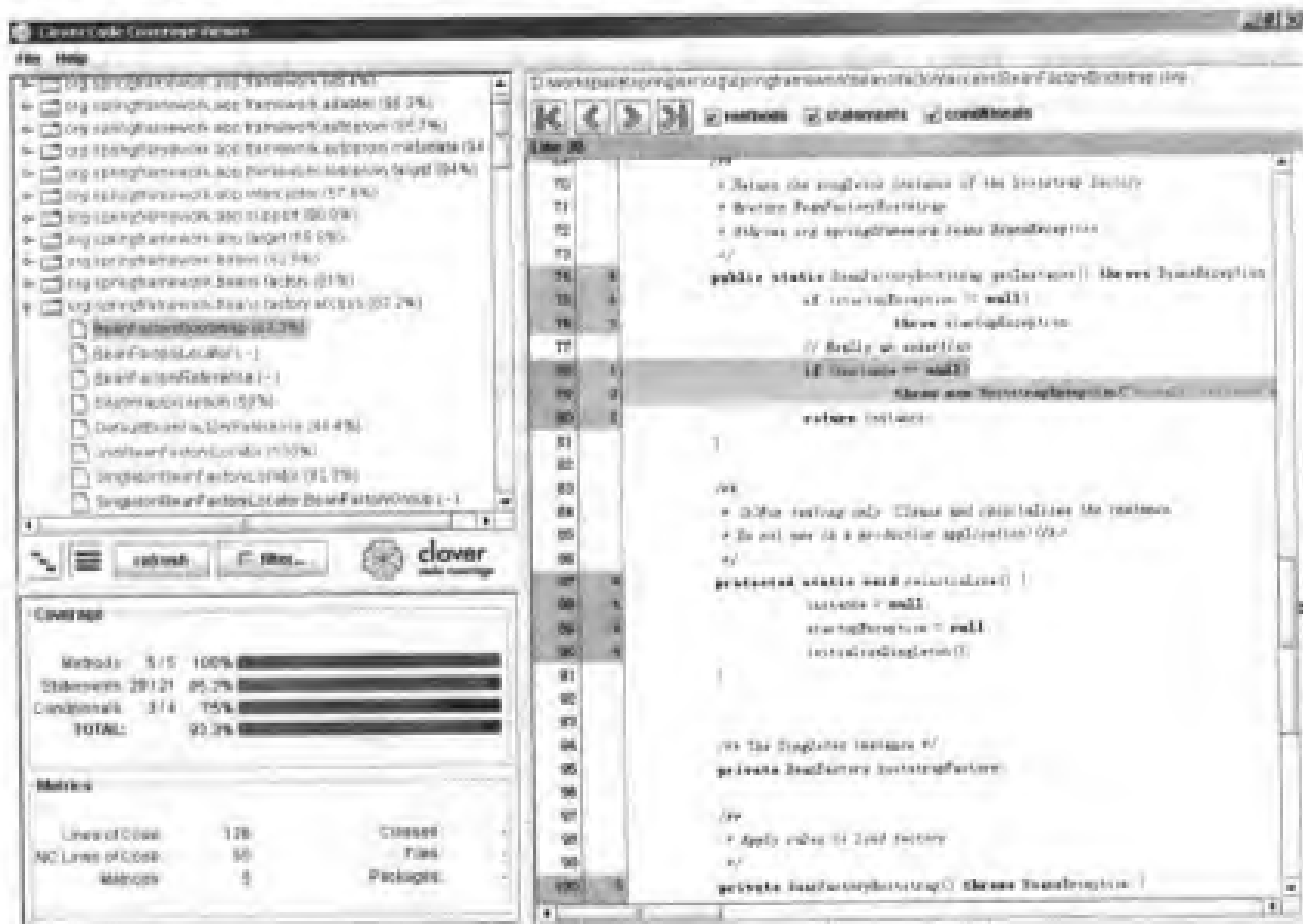
图 2-11 clover.swing 执行结果
