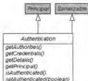
图 17-12 Authentication 接口
