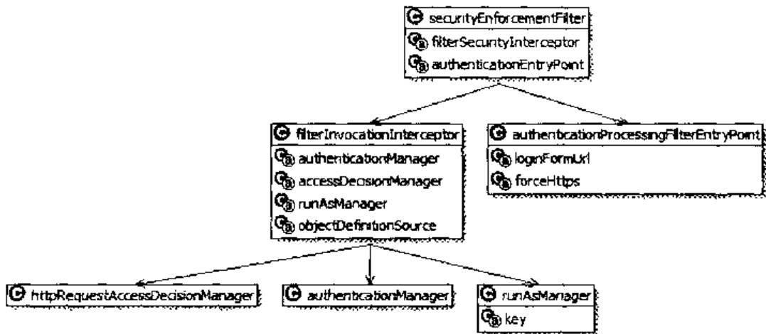
图 17-24 securityEnforcementFilter 过滤器
