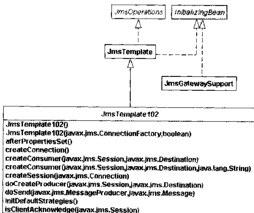
图 8-5 JmsTemplate 和 JmsTemplate102
