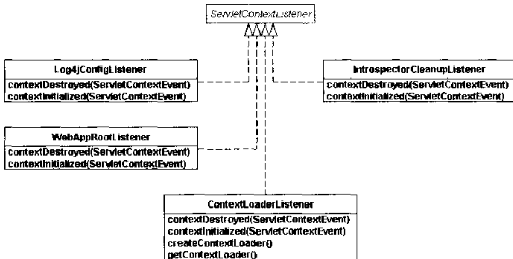
图 3-5 ContextLoaderListener 类图
