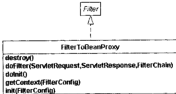
图 17-21 FilterToBeanProxy 过滤器
