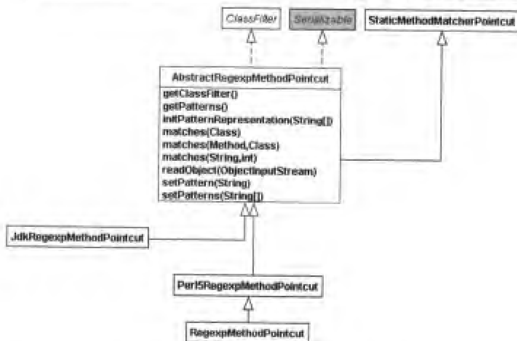
图 4-3 JdkRegexMethodPointcut
