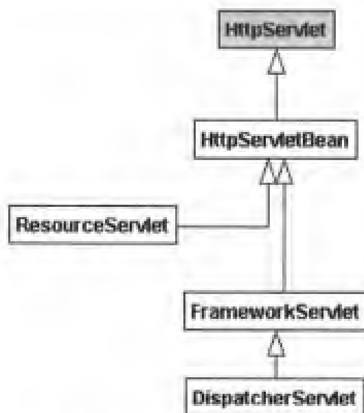
图 14-1 org.springframework.web.servlet.DispatcherServlet 前端控制器
